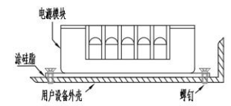
马蹄孔封装安装方式
