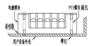
常规安装方式
